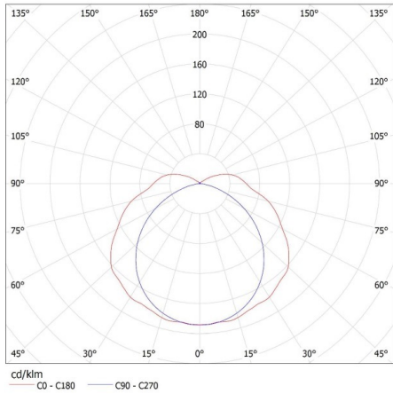
KANLUX S.A. (kat 22801) MAH PLUS-258/4LED/ i GLASSv2 / Krzywa rozsyłu światła (biegunowo) Oprawa: KANLUX S.A. (kat 22801) MAH PLUS-258/4LED/ i GLASSv2 Lampy: 2 x T8 LED GLASSv2 24W-NW
