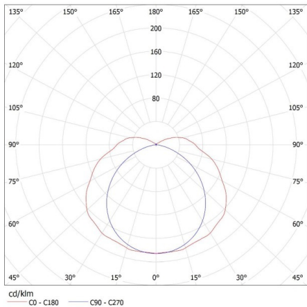
KANLUX S.A. (kat 22801) MAH PLUS-258/4LED/ i T8 Miledo / Krzywa rozsyłu światła (biegunowo) Oprawa: KANLUX S.A. (kat 22801) MAH PLUS-258/4LED/ i T8 Miledo Lampy: 2 x T8 LED 22W-NW
