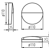
DULI LED 4W-NW-O-GR
