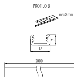
PROFILO B 2M
