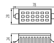
RANGO MINI R7S SMD
