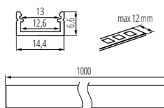
PROFILO J; J-W
