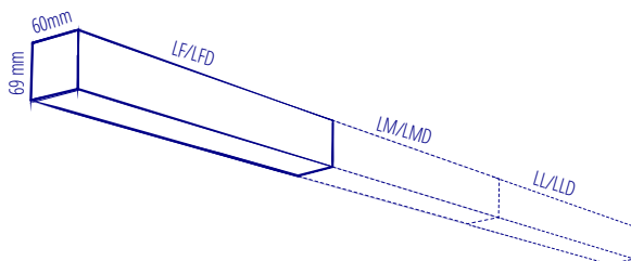
SUSPENSION A SOSPENSIONE
