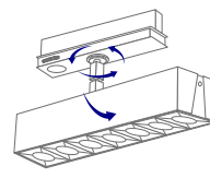
6/ SUR RAIL ORIENTABLE FLEX 340° 90° MONTAGGIO IN SUPERFICIE FLEX ORINTABILE SU DUE ASSI DI 340° E 90°
