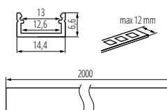
PROFILO J; J-W 2M
