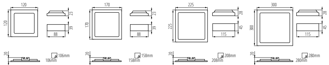
KATRO V2LED 6W
