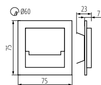
SARIK MINI LED
