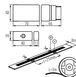
COB SET 3M DIM
