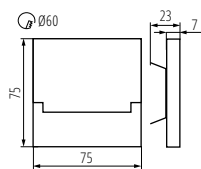
SARIK I ED
