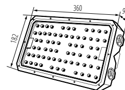
El Stader 200W 60D NW
