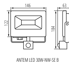
ANTEM LED 30W-NW-SE B
