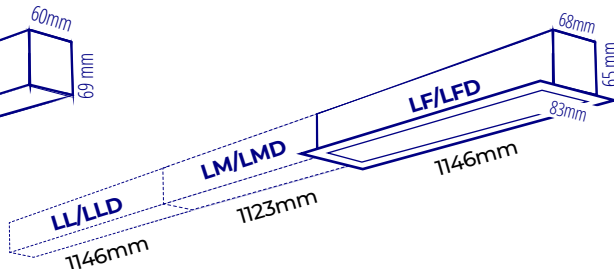
ABMESSUNGEN DER UNTERPUTZVERSION: PT | RECESSED VERSION DIMENSIONS: PT
