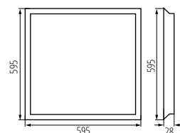
BLINGO UHRA 95 60NW
