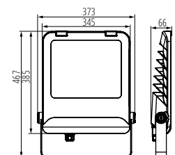
FL AGOR AIO M200W
