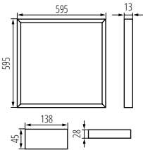
AVAR U 6060 32W-NW
