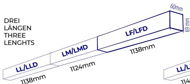
ABMESSUNGEN DER AUFPUTZVERSION: NT | SURFACE VERSION DIMENSIONS: NT
