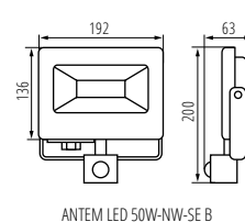
ANTEM LED 50W-NW-SE B
