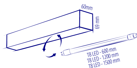
AUFPUTZ SURFACE MOUNTED
