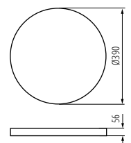
S PLAFON 20W CCTDIM
