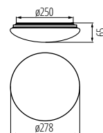
CORSO LED V2 12W / 12W -SE
