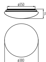
CORSO LED V2 24W / 24W -SE
