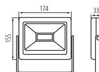
GRUN V3 LED-50-B
