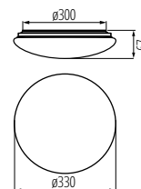
CORSO LED V2 18W / 18W -SE
