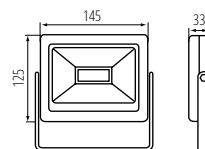
GRUN V3 LED-30-B
