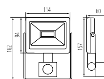
GRUN V3 LED-10-B-SE
