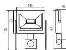
GRUN V3 LED-30-B-SE
