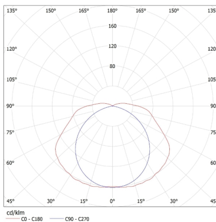
MILED0 (kat 31062) DICHT 4LED N 236/PS i T8 Miledo / LDC (Polar)
