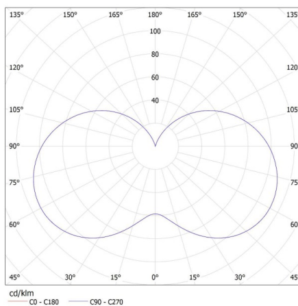
KANLUX S.A. (kat 27297) IQ-LED C37E14 7,5W-WW / LDC (Polar)
