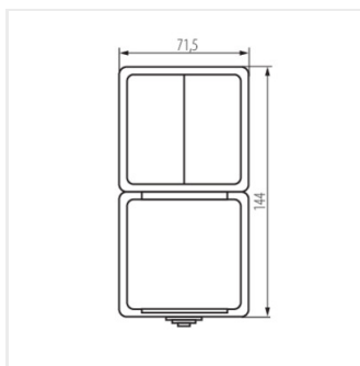
TEKNO 05-3529-143 sz
