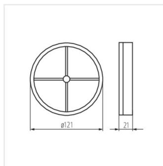
WIR ZL120
