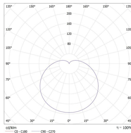
MILED0 (kat 31313) G45 N 6,5W E14-WW / LDC (Polar)
