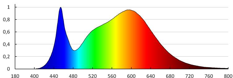
MILED o (kat 31314) G45 N 6,5W E27-NW / LDC (Polar)
