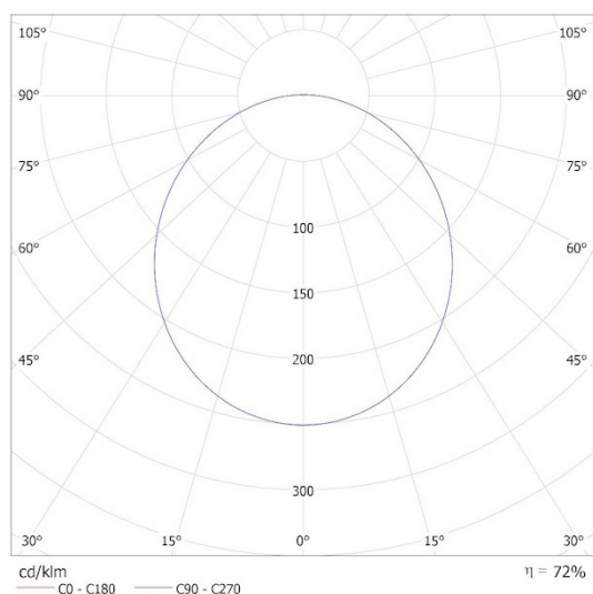
KANLUX S.A. (kat 38777) BENO 12-18W CCT-O-SEW 12W / Krzywa rozsyłu światła (biegunowo)
