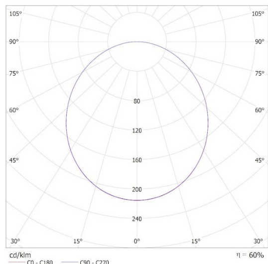
KANLUX S.A. (kat 38779) BENO 24-30W CCT-L G 24W / Krzywa rozsyłu światła (biegunowo)
