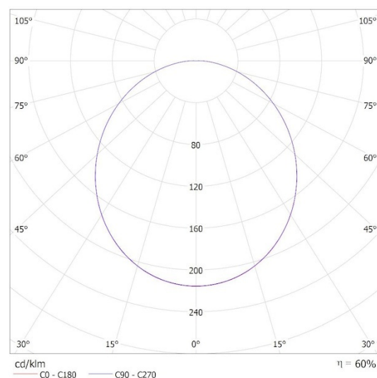
KANLUX S.A. (kat 38780) BENO 24-30W CCT-L-SEG 24W / Krzywa rozsyłu światła (biegunowo)
