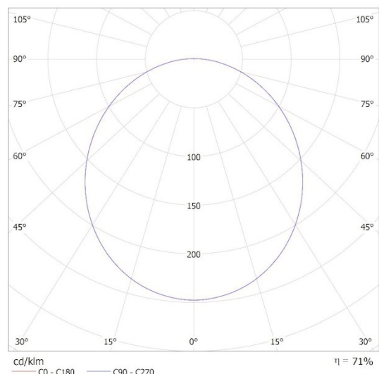
KANLUX S.A. (kat 38782) BENO 24-30W CCT-L W 24W / Krzywa rozsyłu światła (biegunowo)
