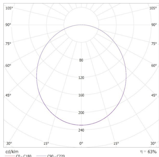
KANLUX S.A. (kat 38783) BENO 24-30W CCT-O G 24W / Krzywa rozsyłu światła (biegunowo)
