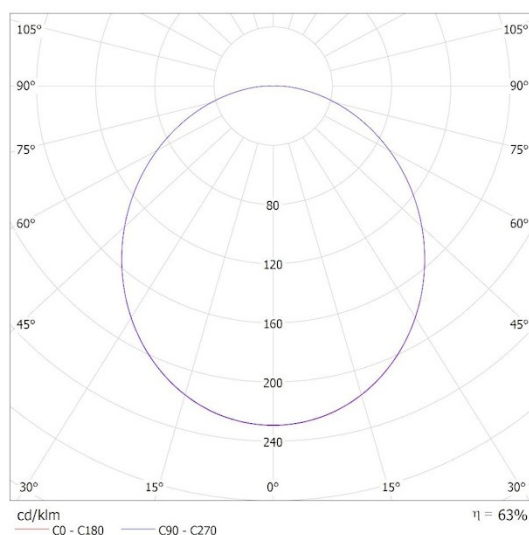
KANLUX S.A. (kat 38784) BENO 24-30W CCT-O-SEG 24W / Krzywa rozsyłu światła (biegunowo)
