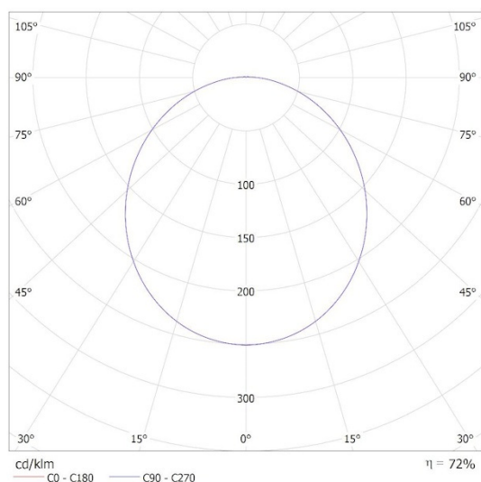
KANLUX S.A. (kat 38785) BENO 24-30W CCT-O-SEW 24W / Krzywa rozsyłu światła (biegunowo)
