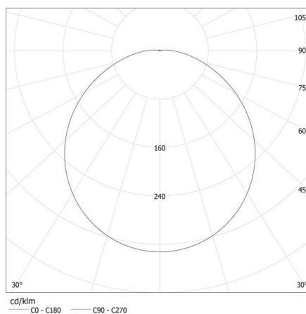
KANLUX S.A. (kat 18121) FOGLER LED 14W-NW / Krzywa rozsyłu światła (biegunowo)
