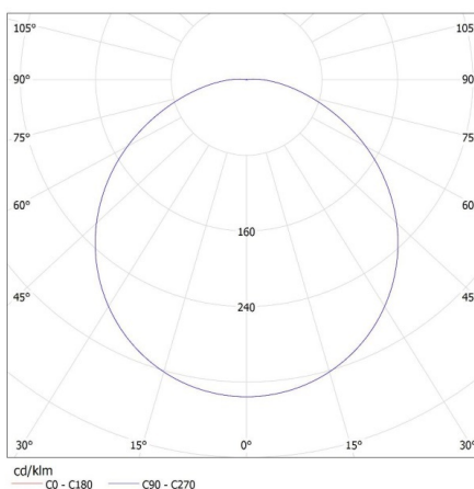
KANLUX S.A. (kat 19064) DABA PRO 25W NW-W / LDC (Polar)
