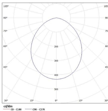
KANLUX S.A. (kat 19760) GAVI LED18 SMD / Krzywa rozsyłu światła (biegunowo)
