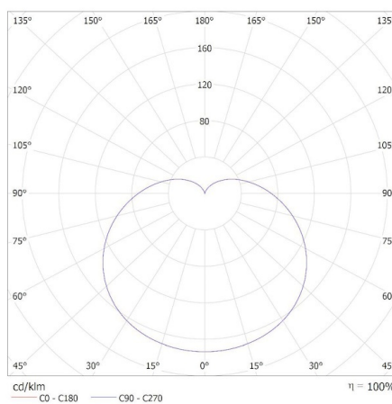
KANLUX S.A. (kat 26766) BILO 6,5W E14-NW / Krzywa rozsyłu światła (biegunowo)
