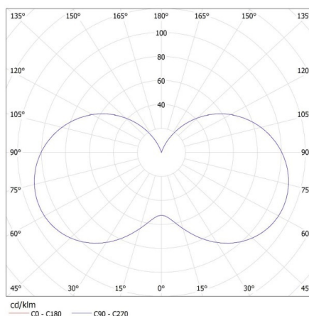
KANLUX S.A. (kat 27295) IQ-LED C37E14 5,5W-NW / LDC (Polar)
