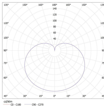
KANLUX S.A. (kat 27313) IQ-LED A67 17,5W-NW / LDC (Polar)
