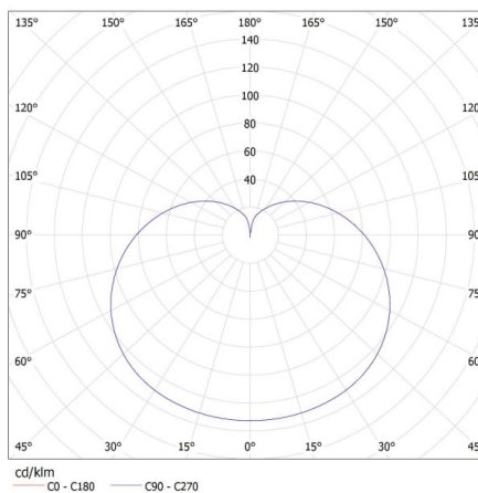
KANLUX S.A. (kat 27317) IQ-LED A67 19W-CW / LDC (Polar)
