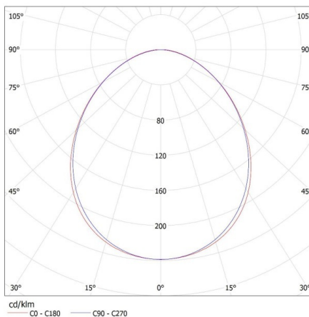
KANLUX S.A. (kat 27423) ALIN 4LED 1X150-B + GLASSv4 / LDC (Polar)
