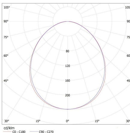
KANLUX S.A. (kat 27423) ALIN 4LED 1X150-B + GLASSv3 / LDC (Polar)
