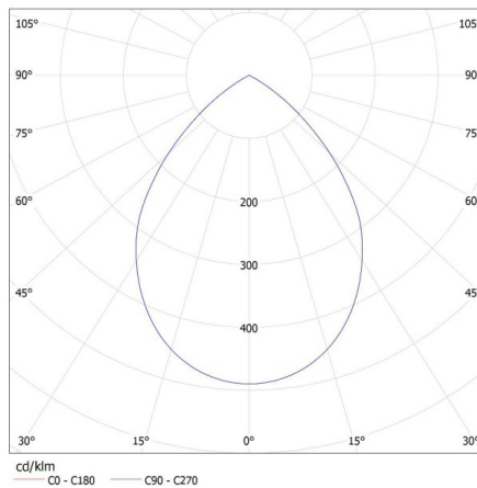
KANLUX S.A. (kat 27571) RITI GU10 B/G + TOMI LED5W / LDC (Polar)
