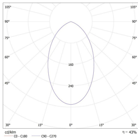
KANLUX S.A. (kat 29237) GOVIK ST DSO-B + IQ-LED ... 7W S3 / LDC (Polar)
