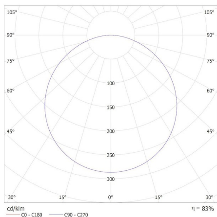
KANLUX S.A. (kat 29816) BLINGO R 36W 6060 WW / Krzywa rozsytu światła (biegunowo)
