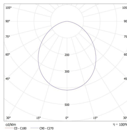
MILED0 (kat 31233) GU10 6W-WW LED / LDC (Polar)
