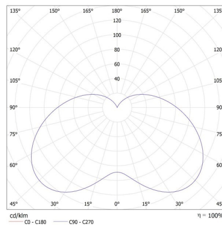
MILEDO (kat 31308) C35 N 6,5W E14-NW / LDC (Polar)
