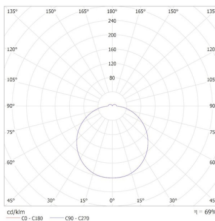
MILED0 (kat 31491) TURA LED 24W-NW-O-B / Krzywa rozsyłu światła (biegunowo)
