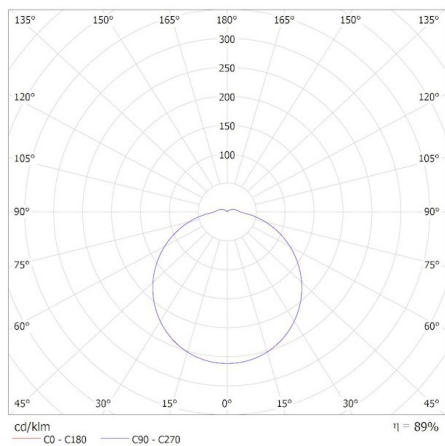
Miledo (kat 31498) TOLU O LED 18W-NW-W / Krzywa rozsyłu światła (biegunowo)
