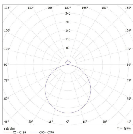
MILED0 (kat 31501) AZPO LED 11,8W-NW-O-B / Krzywa rozsyłu światła (biegunowo)
