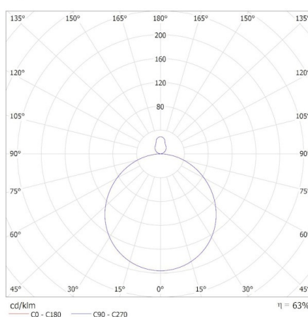
MILED0 (kat 31504) AZPO LED 22W-NW-O-W / Krzywa rozsyłu światła (biegunowo)
