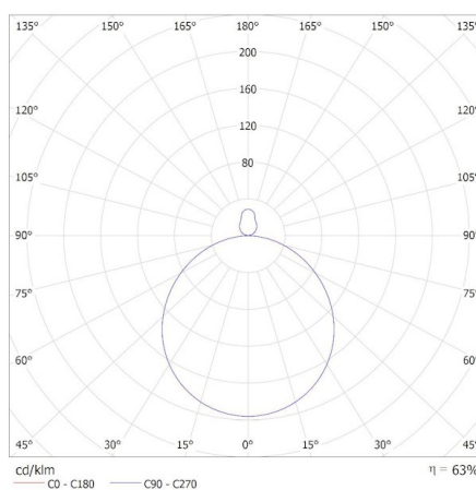
MILED0 (kat 31505) AZPO LED 22W-NW-O-B / Krzywa rozsyłu światła (biegunowo)
