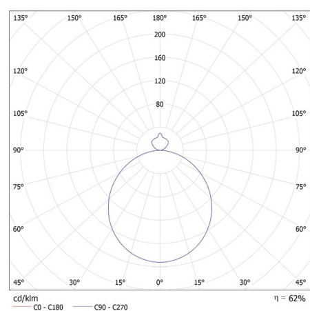
MILED0 (kat 31507) AZPO LED 12,3W-NW-L-B / Krzywa rozsyłu światła (biegunowo)
