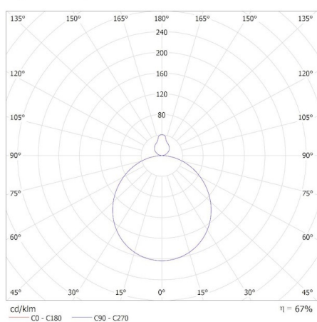
MILED0 (kat 31508) AZPO LED 17,5W-NW-L-W / Krzywa rozsyłu światła (biegunowo)
