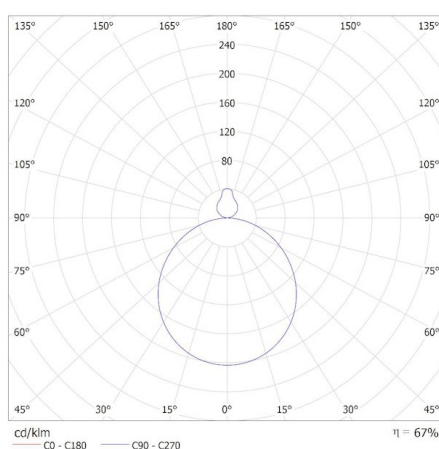
MILED0 (kat 31509) AZPO LED 17,5W-NW-L-B / Krzywa rozsyłu światła (biegunowo)
