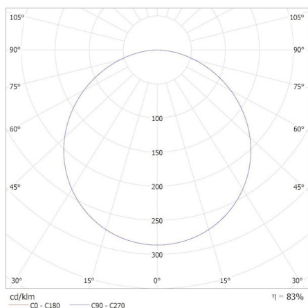
KANLUX S.A. (kat 33174) BLINGO IPRN38W 6060 NW / Krzywa rozsytu światła (biegunowo)
