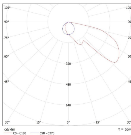
KANLUX S.A. (kat 33694) GLASI LED 3W P NW-B / LDC (Polar)
