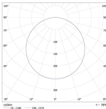
KANLUX S.A. (kat 35002) STIVI LED 36W-NW-O / LDC (Polar)
