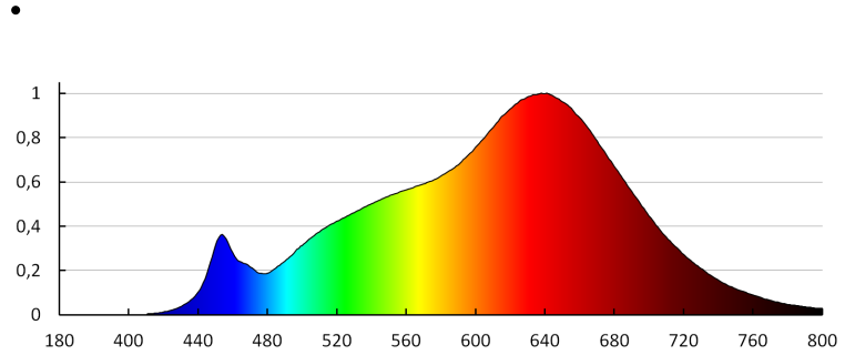
KANLUX S.A. (kat 35252) IQ-LED AR-111 13W-WW / LDC (Polar)
