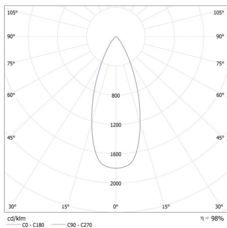
KANLUX S.A. (kat 35280) ELICEO DSO B/B + IQ-LED ... 6,5WS3 / LDC (Polar)
