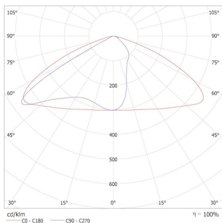
KANLUX S.A. (kat 36229) STRETON LED 40W NW / Krzywa rozsytu światła (biegunowo)
