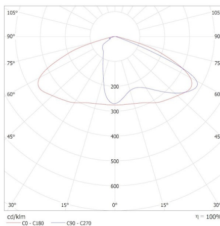
KANLUX S.A. (kat 36232) STRETON LED 150W NW / Krzywa rozsyłu światła (biegunowo)
