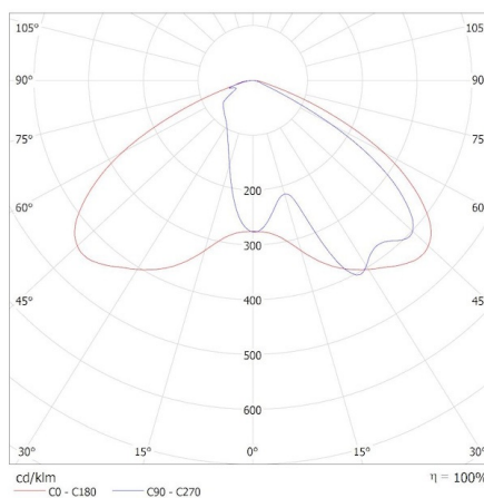
KANLUX S.A. (kat 36233) STRETON LED 200W NW / Krzywa rozsyłu światła (biegunowo)
