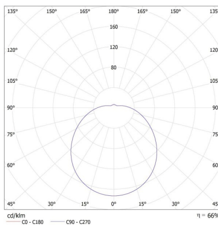
KANLUX S.A. (kat ) RIFA LED 17,5W WW / LDC (Polar)
