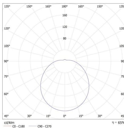
KANLUX S.A. (kat ) RIFA LED 17,5W NW / LDC (Polar)
