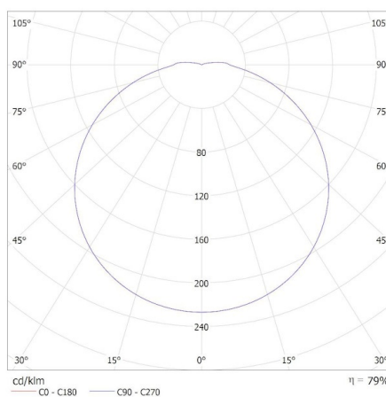
KANLUX S.A. (kat 37299) IPER LED 19W-NW-O-SE / Krzywa rozsyłu światła (biegunowo)
